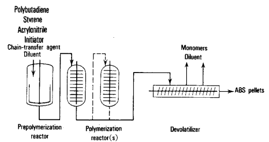
Fig. 4. 연속-괴상중합 공정도.
