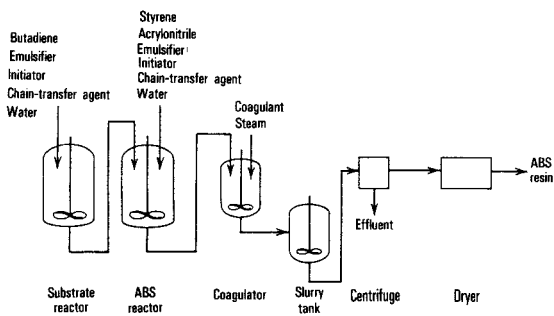
Fig. 2. 유화그라프트중합 공정도.
